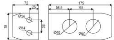
FODL-04 Door Lock (Key & Knob) ₹ 6200.00
