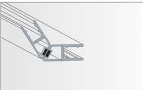
FOGP-M2 135° 8mm (2.2mtr.) ₹ 515.00 8mm (2.5mtr.) ₹ 645.00 10mm (2.2mtr.) ₹ 575.00 10mm (2.5mtr.) ₹ 645.00 12mm (2.2mtr.) ₹ 565.00 12mm (2.5mtr.) ₹ 705.00
