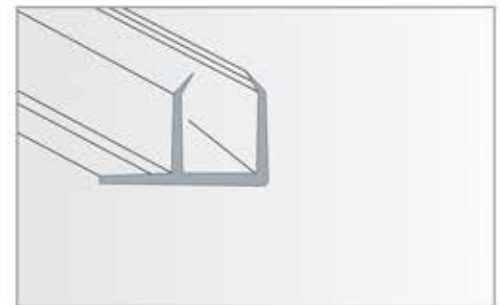
FOGP-6 8mm (2.2mtr.) ₹ 105.00 8mm (2.5mtr.) ₹ 115.00 10mm (2.2mtr.) ₹ 105.00 10mm (2.5mtr.) ₹ 115.00 12mm (2.2mtr.) ₹ 115.00 12mm (2.5mtr.) ₹ 130.00
